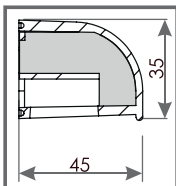
СЕЧЕНИЕ OZ 400
